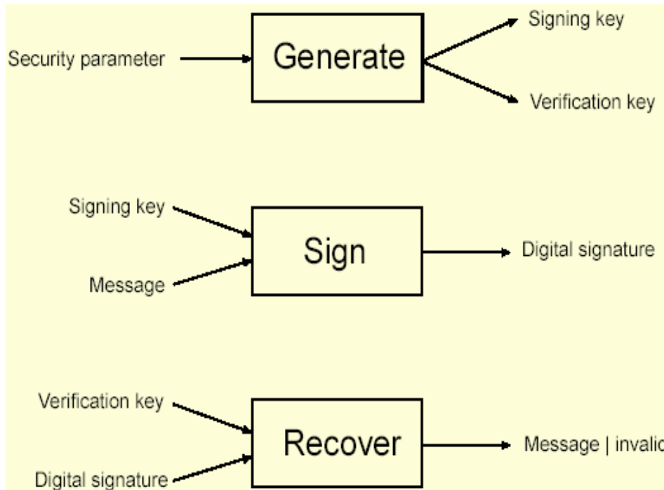
شکل ب-۲-۳: الگوریتم
